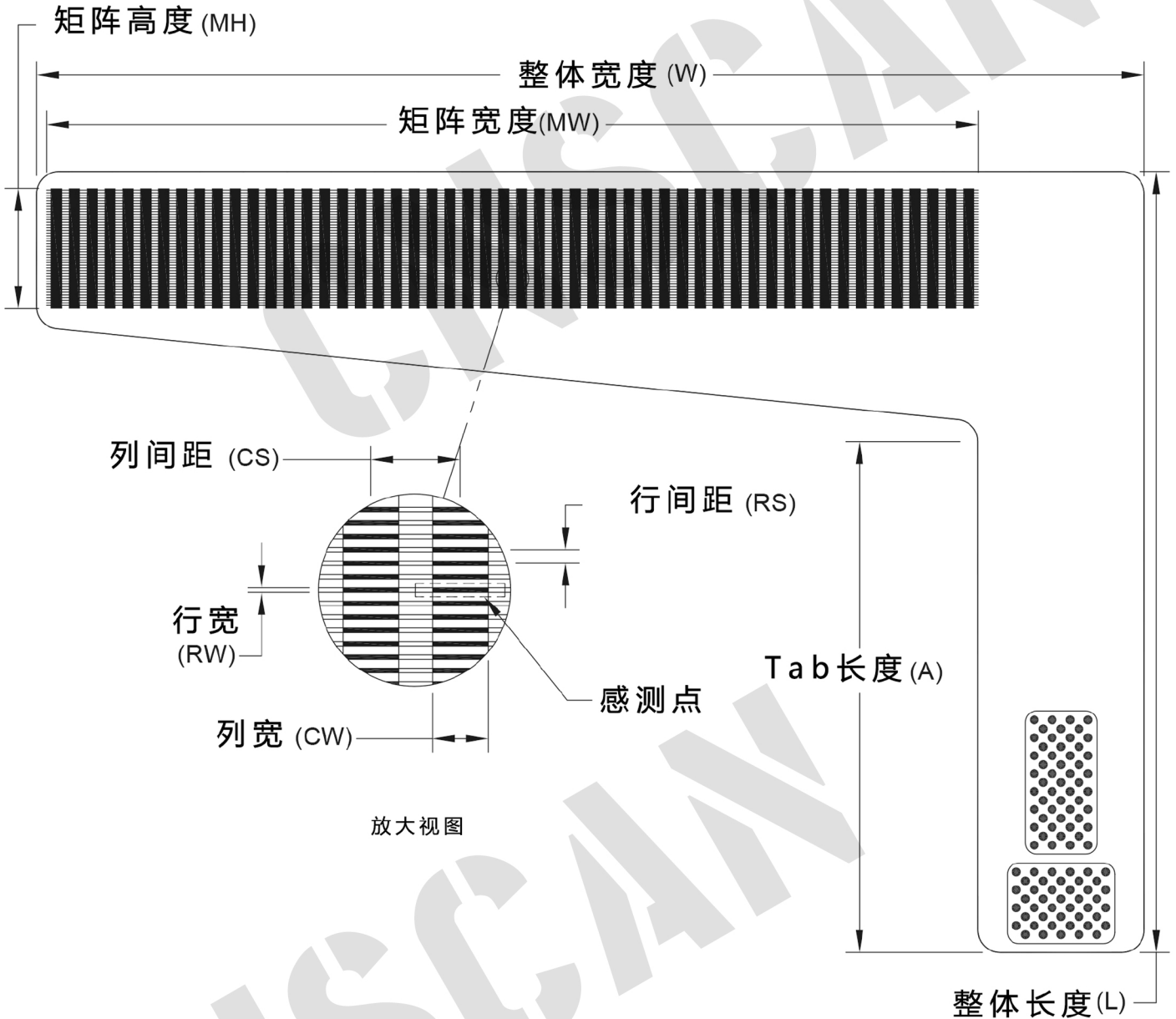
外形尺寸
