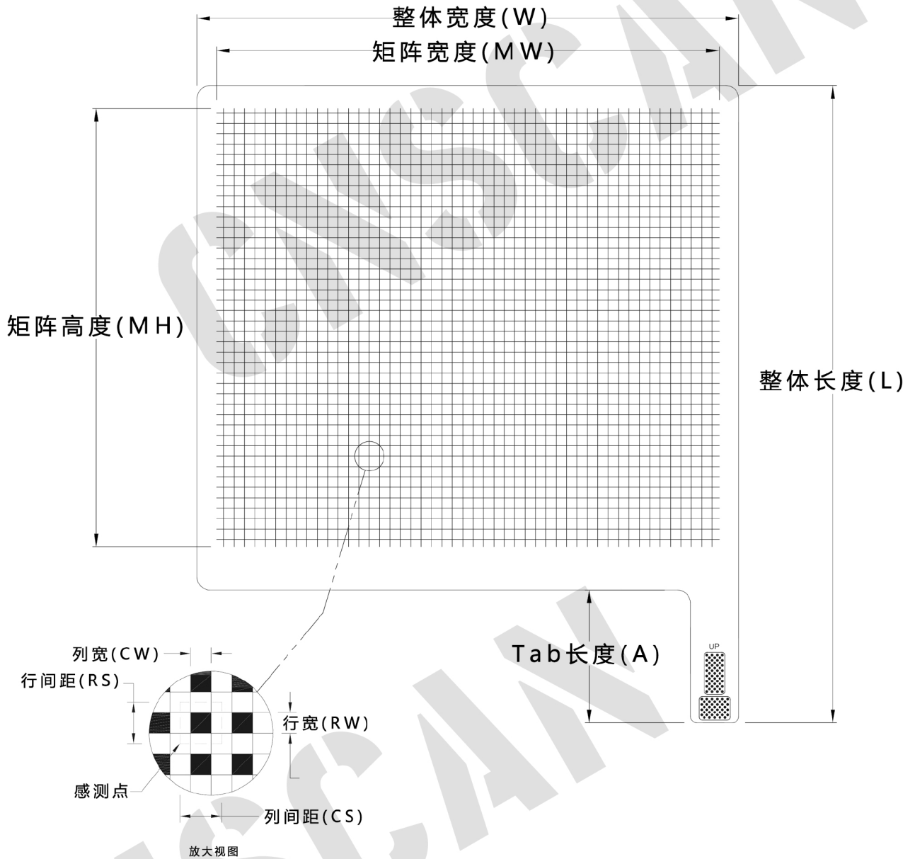
外形尺寸
