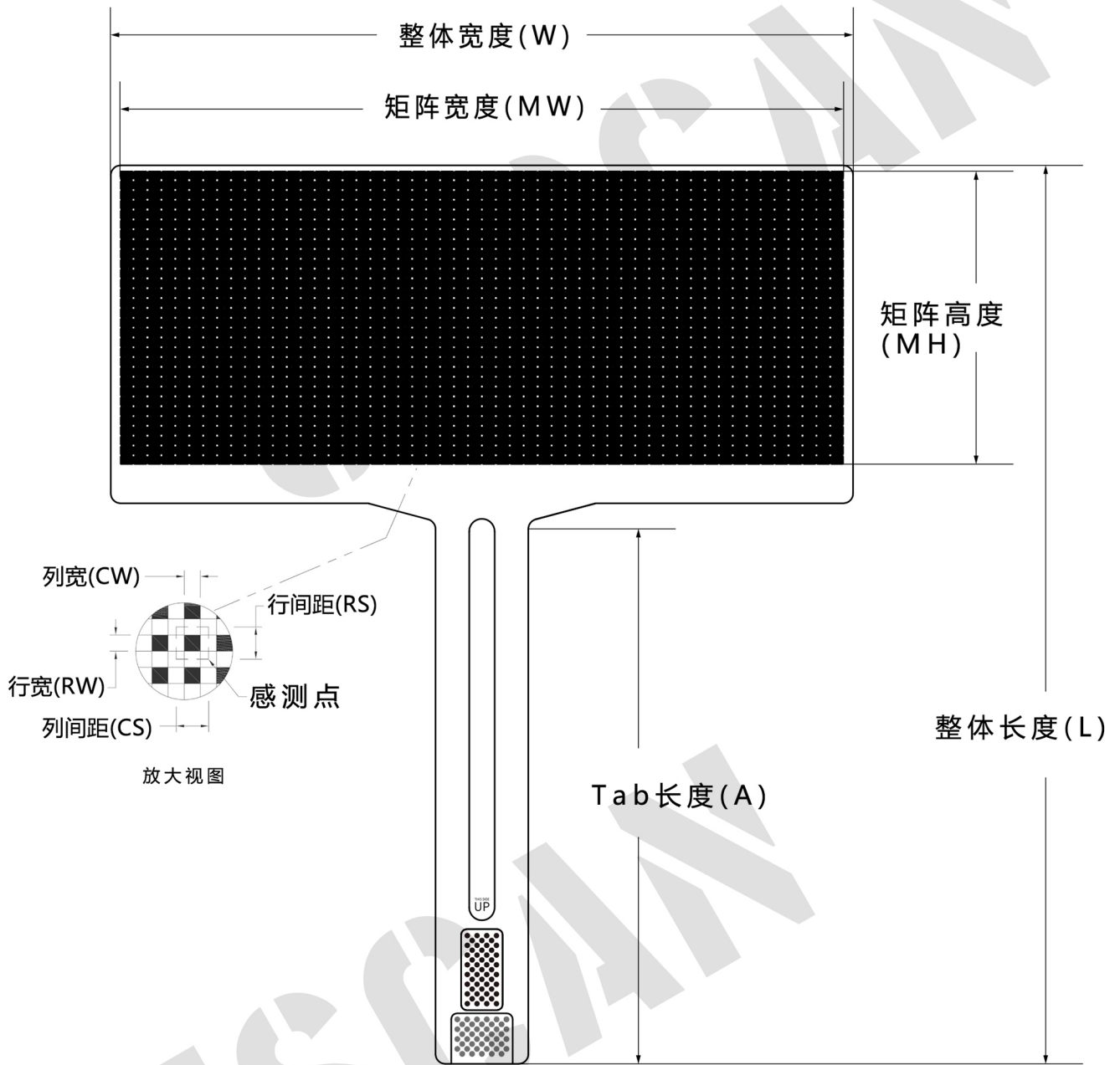
外形尺寸
