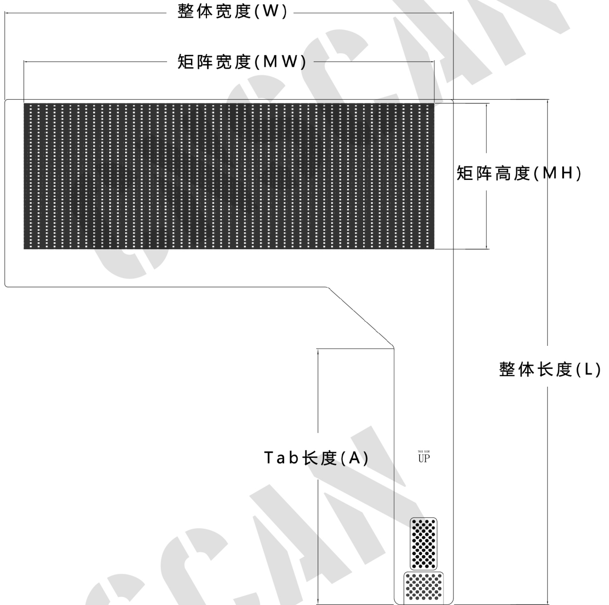
传感区参数
