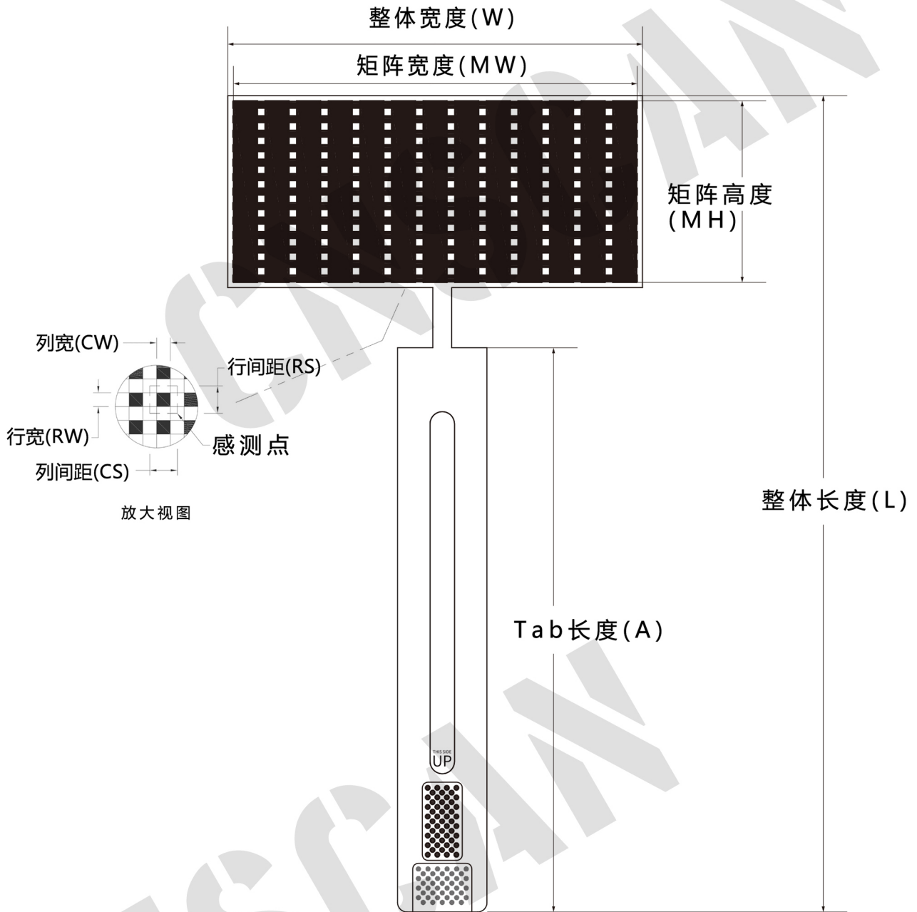
外形尺寸
