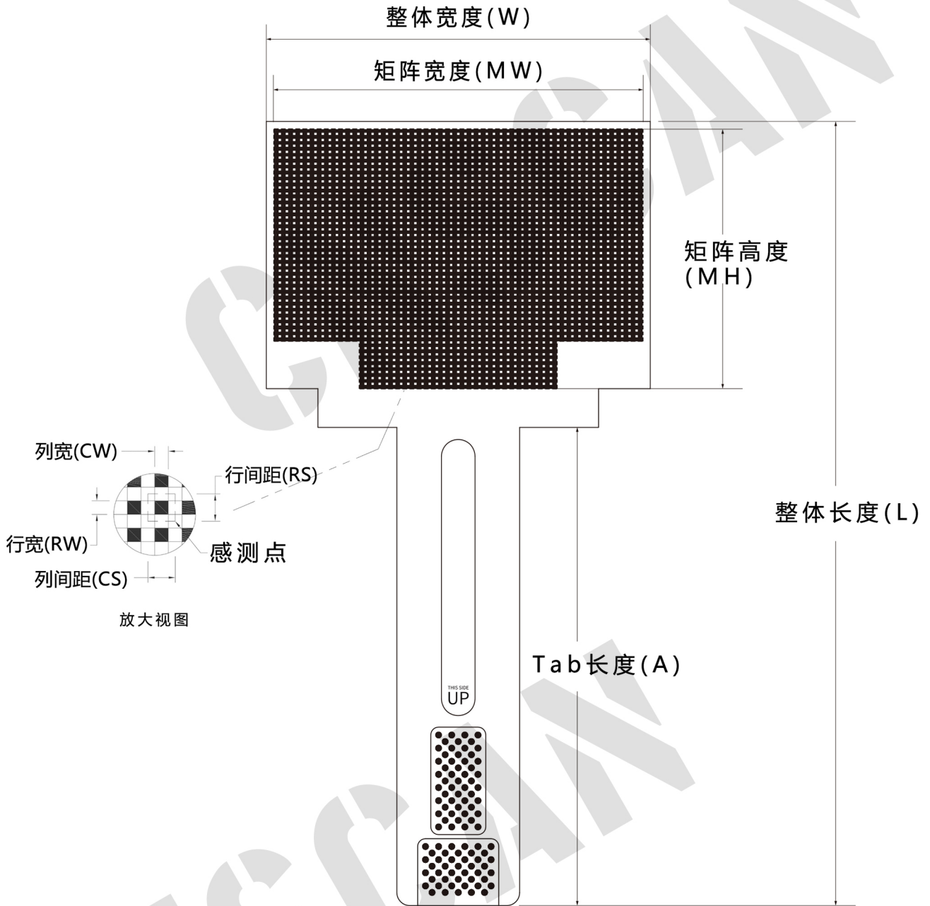
外形尺寸
