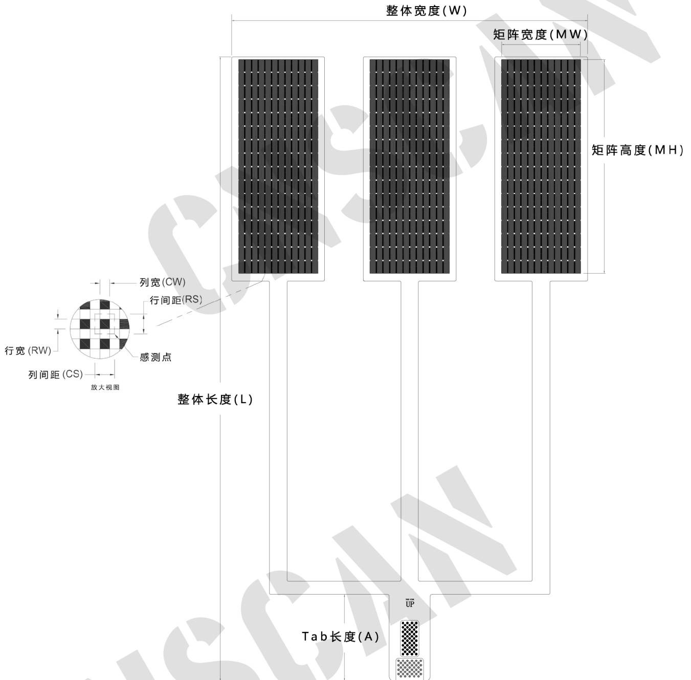
外形尺寸
