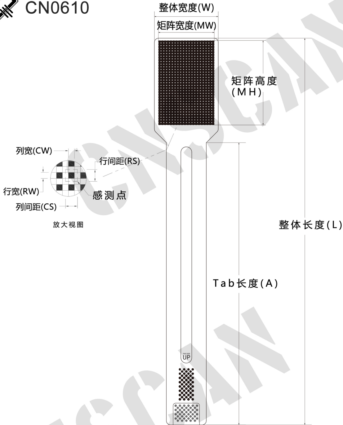
外形尺寸
